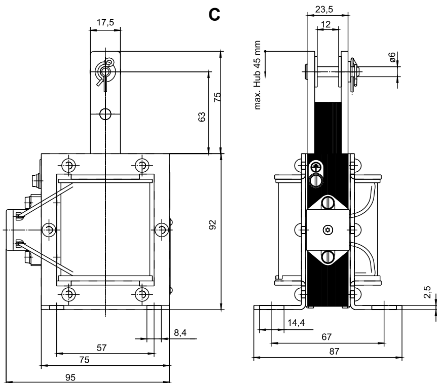
Fig. 5: Type W BA X 070 C00 A01 to W BA X 070 C00 A01 (pull type)
