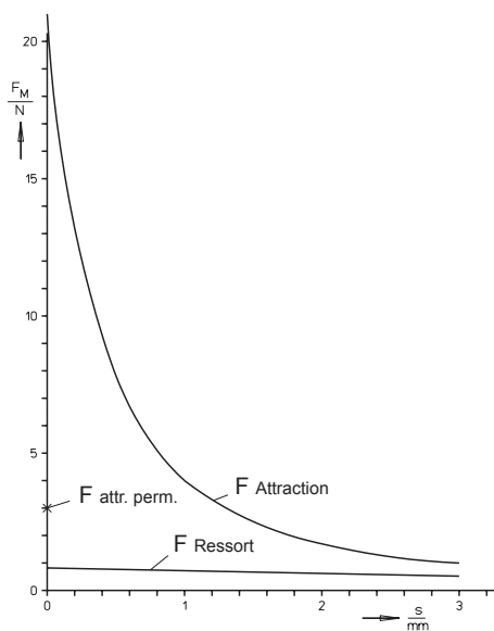
Fig. 3: Courbe caractéristique force / course G BK P 017 K00 A01
